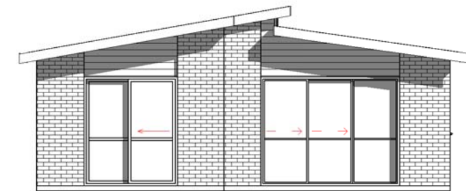
E East 1 : 100
