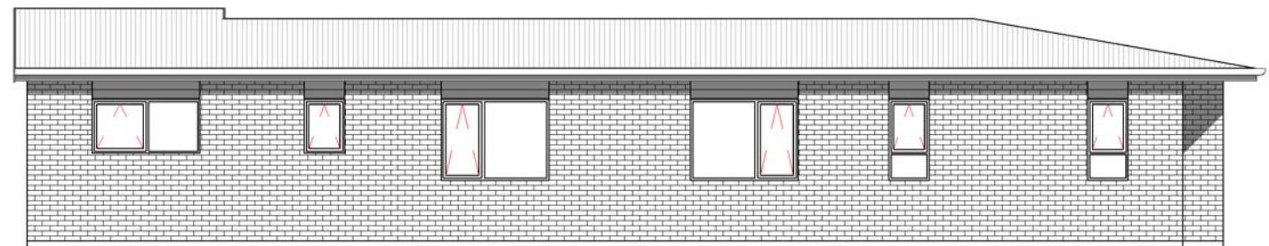
N North 1 : 100
